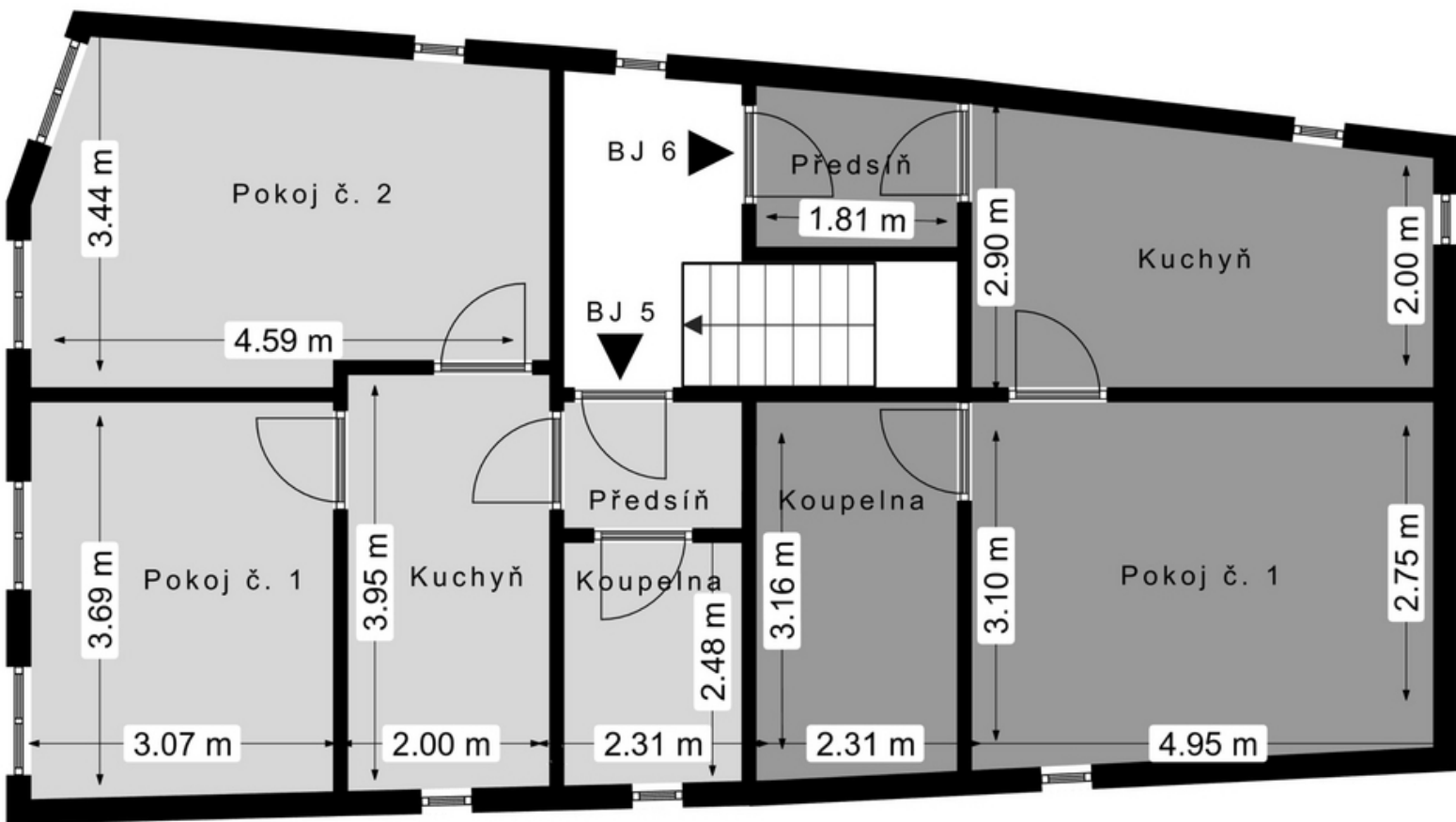
DŮM NA HRADĚ MAHLEROVA 241/13, OLOMOUC 3 NP
