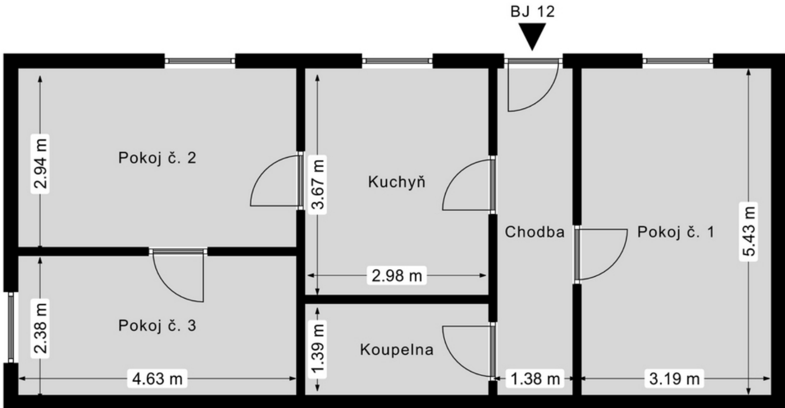
DŮM U HŘIŠTĚ TVRDÍKOVA 65/8, OLMOUC PŘÍZEMÍ
