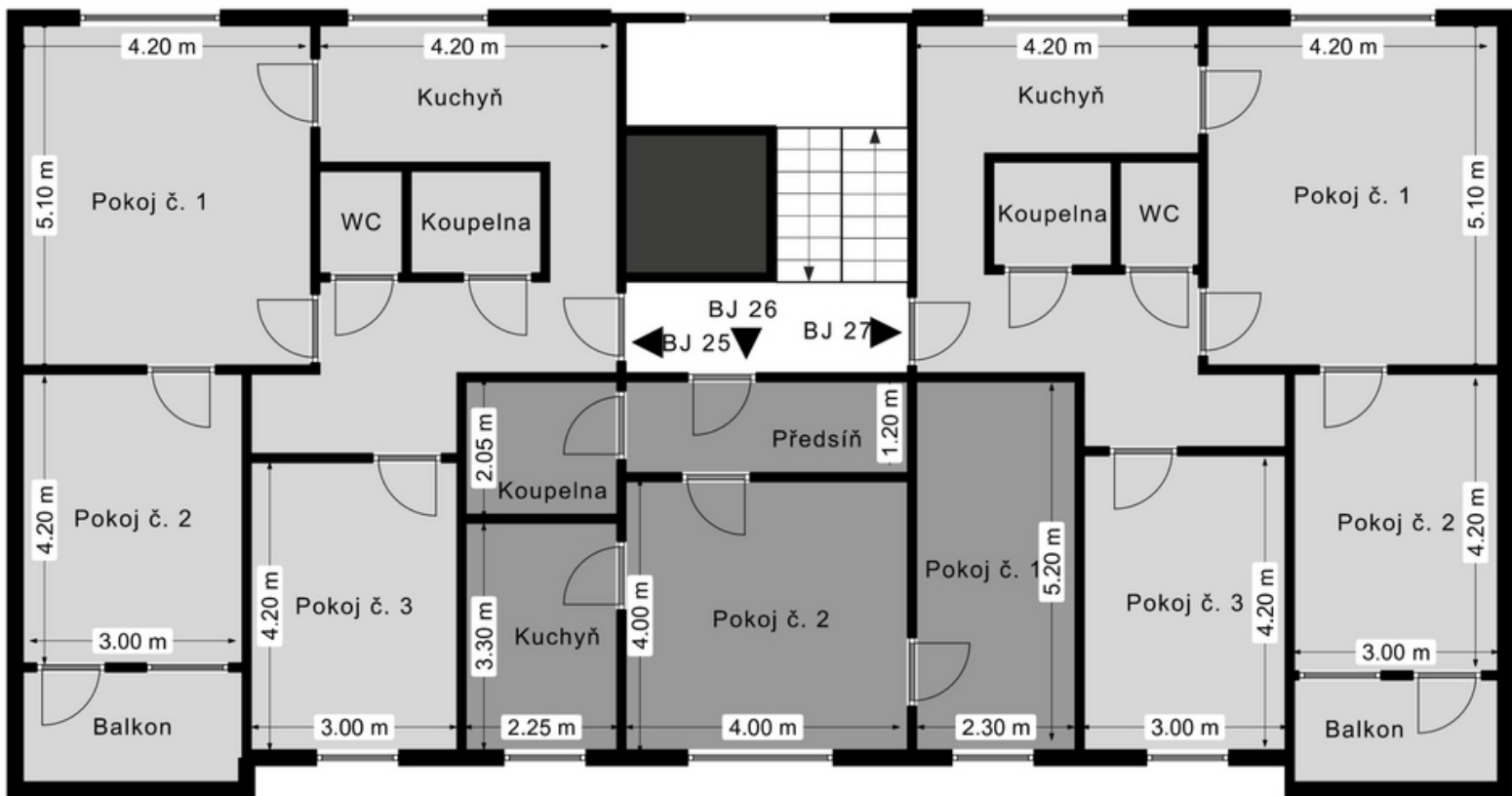
DŮM U ŘEKY ROKYCANOVA 519/7, OLMOUC 2 NP
