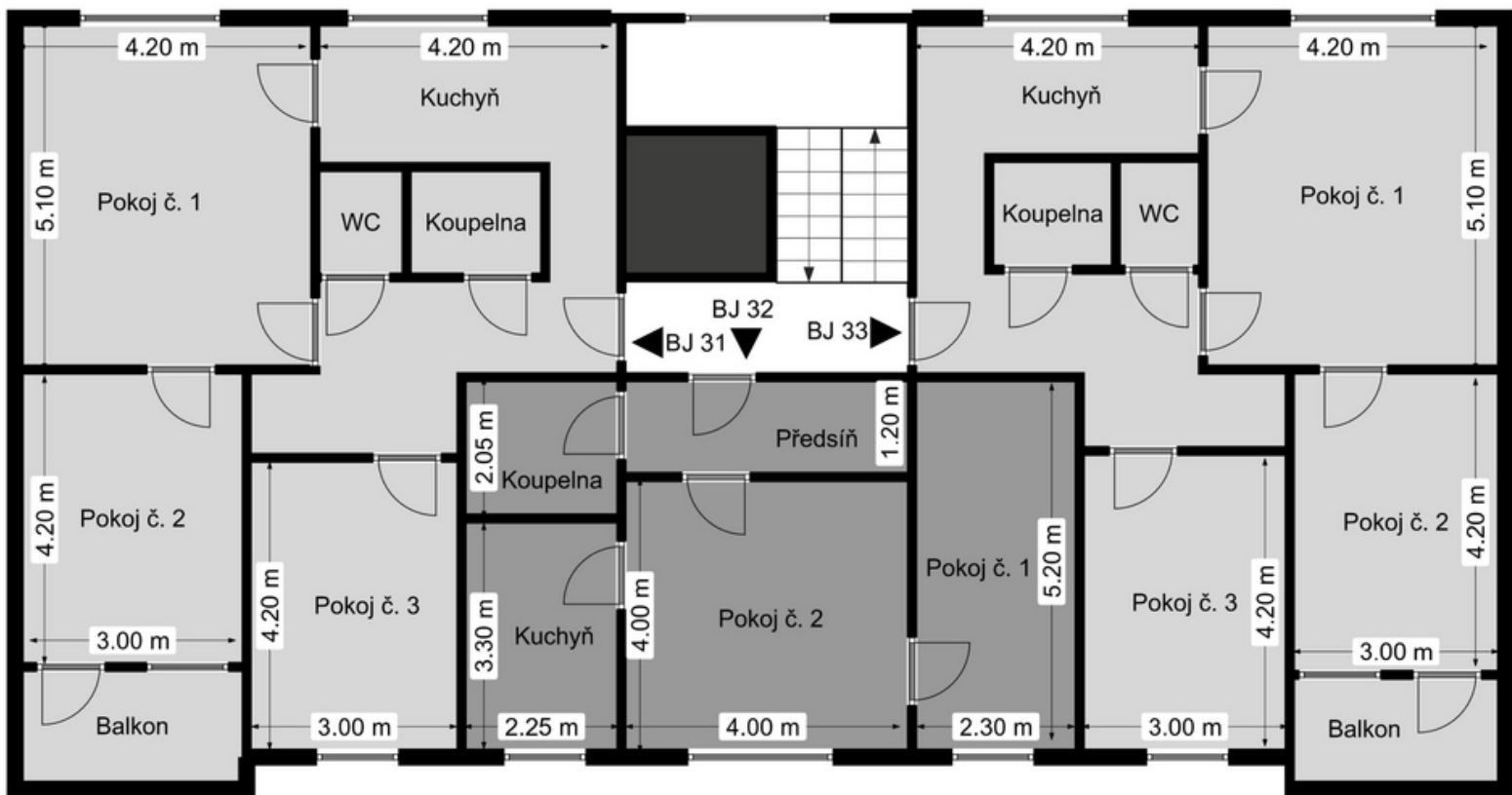
DŮM U ŘEKY ROKYCANOVA 519/7, OLMOUC 4 NP
