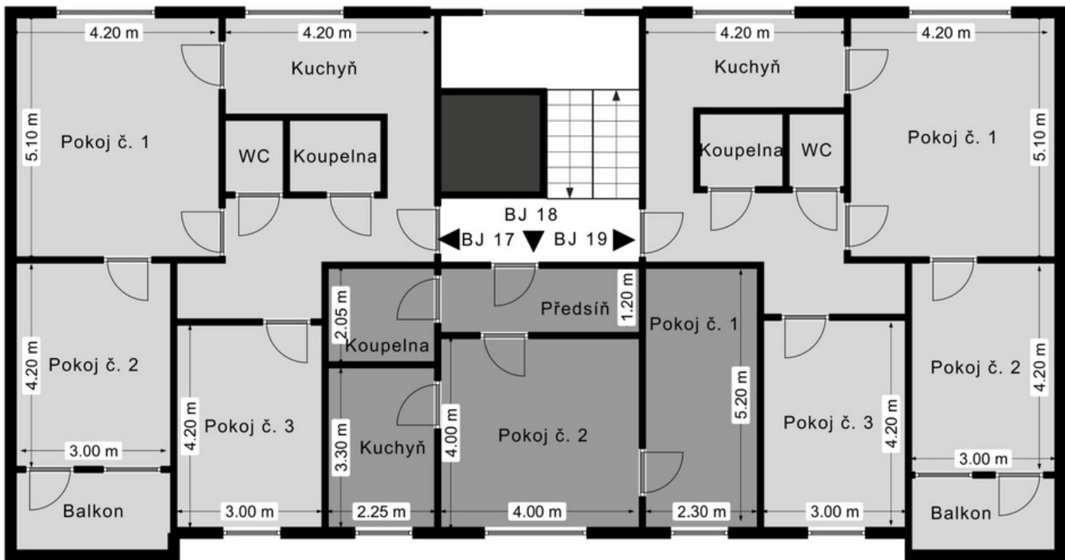
DŮM U ŘEKY ROKYCANOVA 518/5, OLMOUC 3 NP
