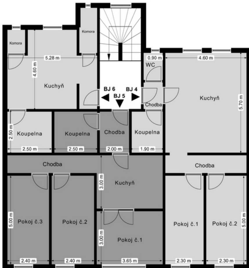
BYTOVÝ DŮM TŘINÁCTKA TŘÍDA SVORNOSTI 147/13, OLMOUC 2 NP
