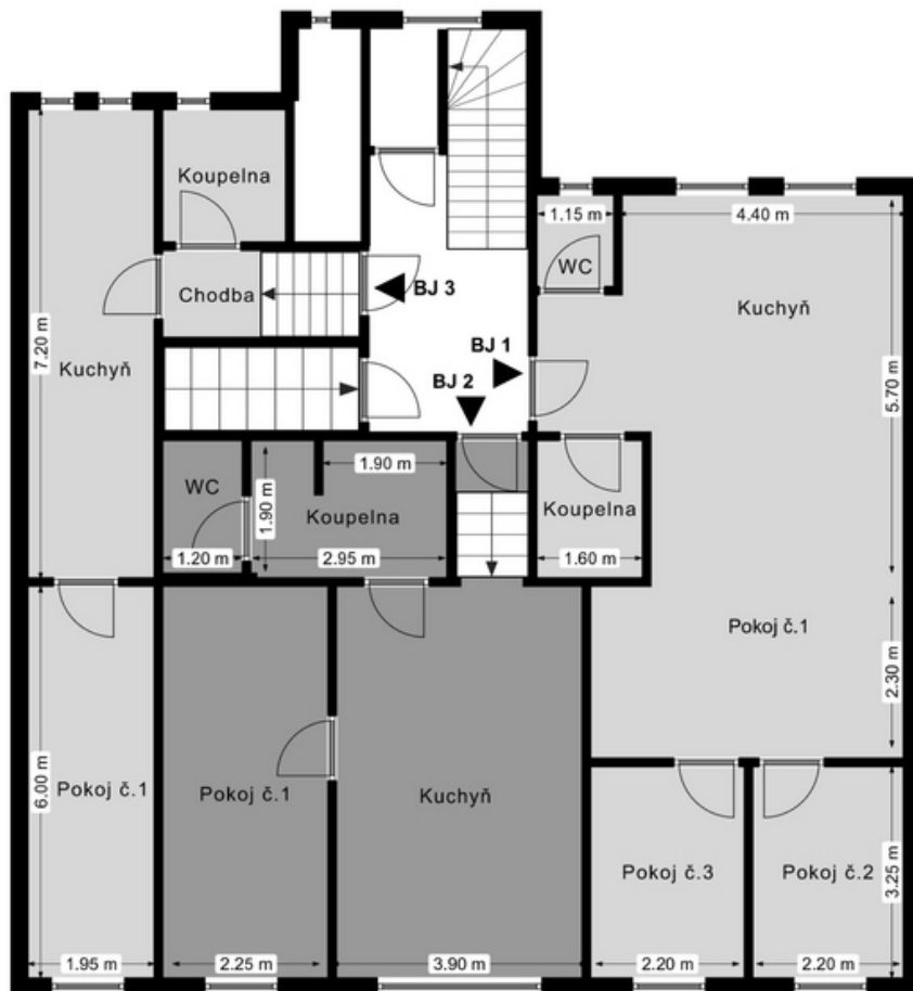
BYTOVÝ DŮM TŘINÁCTKA TŘÍDA SVORNOSTI 147/13, OLOMOUČ 1 NP
