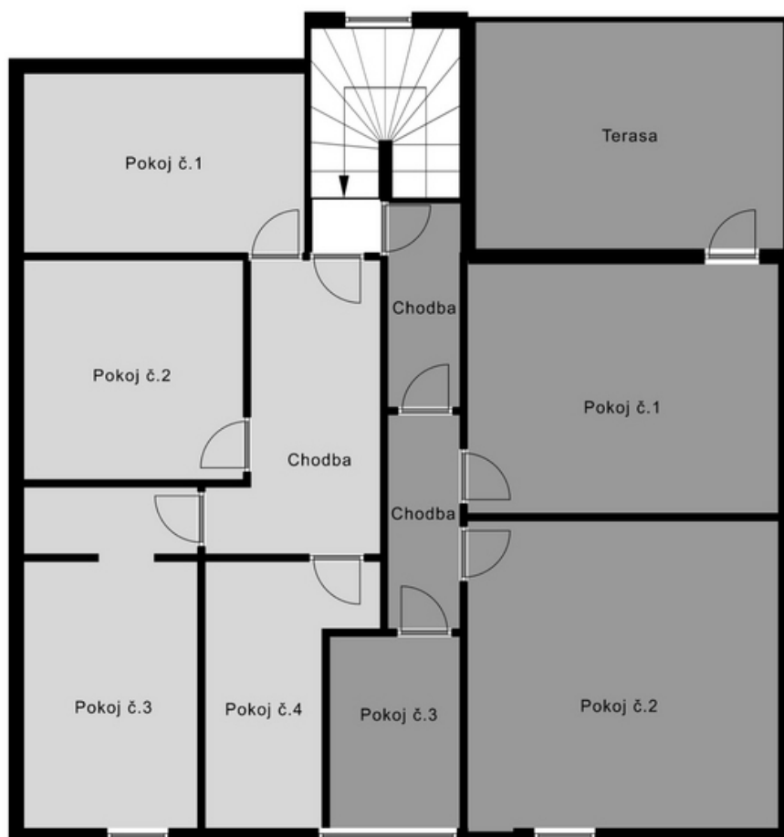
BYTOVÝ DŮM TŘINÁCTKA TŘÍDA SVORNOSTI 147/13, OLOMOUC 4 NP - PODKROVÍ
